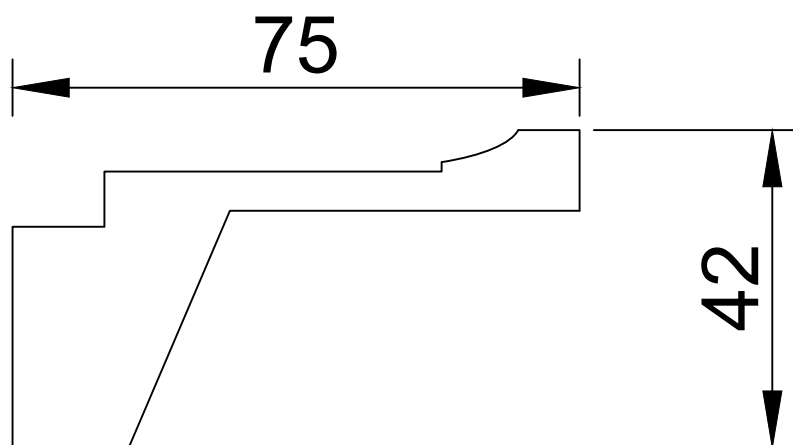
Side Scale 1:1
