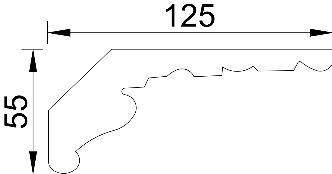
Side Scale 1:1
